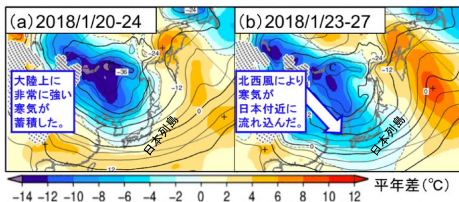
【図 1 上空 1,500m の気温分布図：気象庁 HP より】
